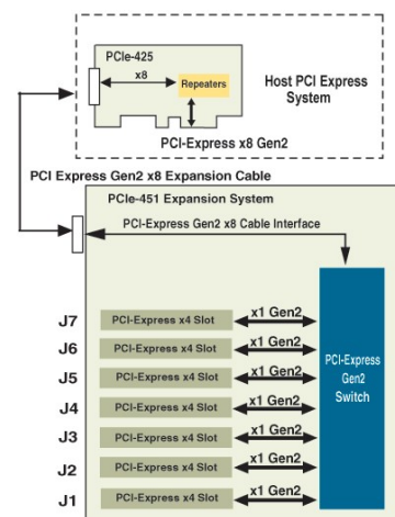
構成図
