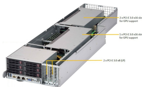
PCI-Express3.0 バス配置
